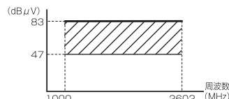
図1. 入力レベル上限値
